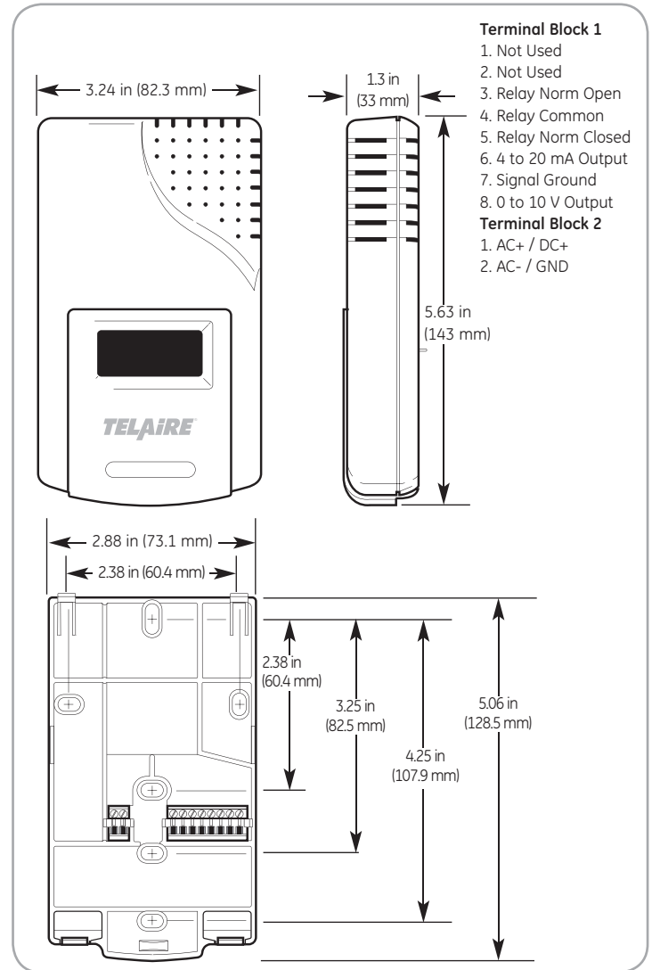
Ventostat 8200-ACD Dimensions
